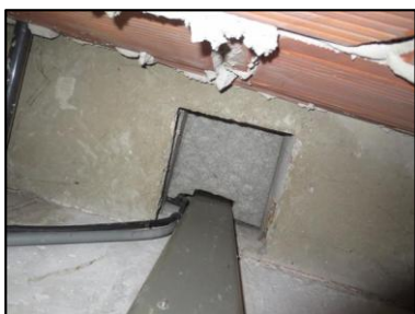
Photo N° 1141 AMIANTE CIMENT - -placards technique rdc à +9 Planchers Plaques planes (Fibres- ciment)
